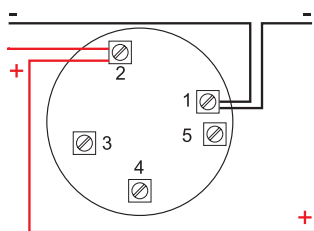
Base LPB conectada a AWS32/R (sirena sin aislador)
