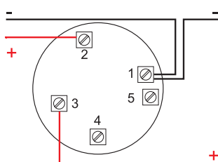
Base LPB conectada a AWS32/R-I (sirena con aislador)
