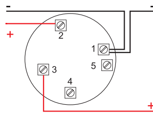
Base LPB conectada a ABS32/W-I (sirena con aislador)
