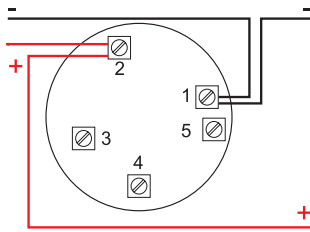
Base LPB conectada a ABS32/W (sirena sin aislador)
