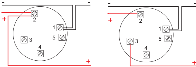
Base LPB conectada a ABSB32/W/C (sirena sin aislador)
